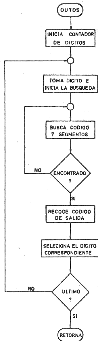
Fig. - 13 RUTINA DE REFresco DEL VISUALIZADOR
