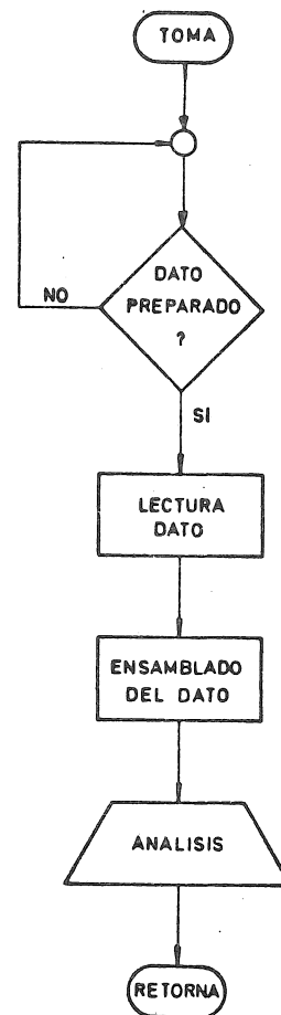
Fig. - 9 PROGRAMA DE TOMA DE DATOS
