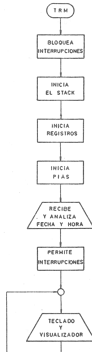
Fig. _ 7 PROGRAMA DE PREPARACION DE LA OPERACION DEL SISTEMA
