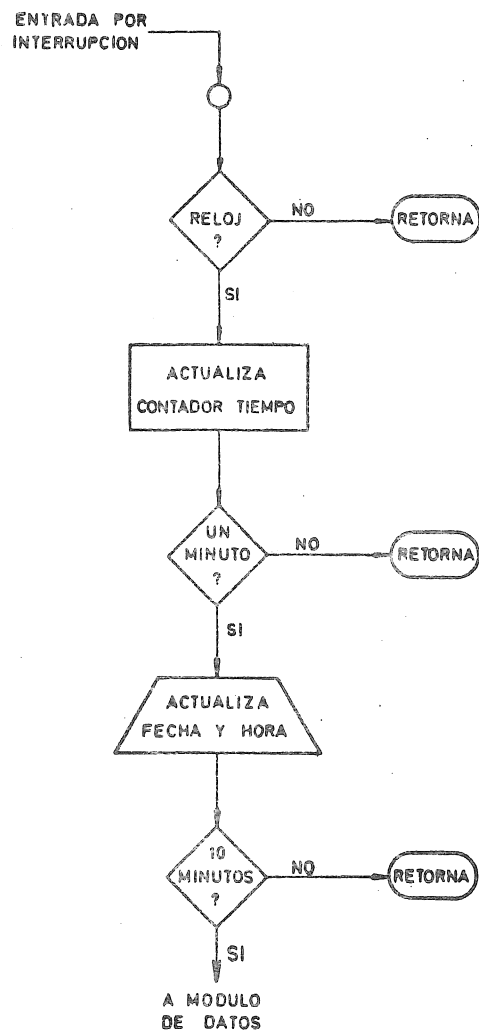
Fig. - 8 RUTINA DE SERVICIO AL RELOJ
