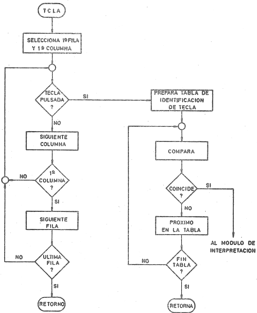
Fig. 14 RUTINA DE ESCRUTADO DEL TECLADO
