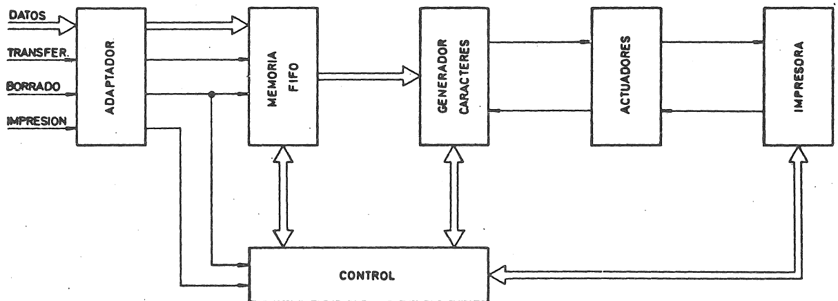
Fig. _ 2 CONTROL DE LA IMPRESORA
